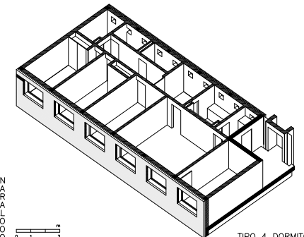
TIPO 4 DORMITORIOS
