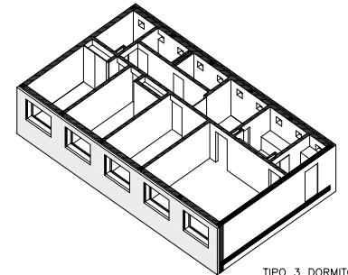
TIPO 3 DORMITORIOS
