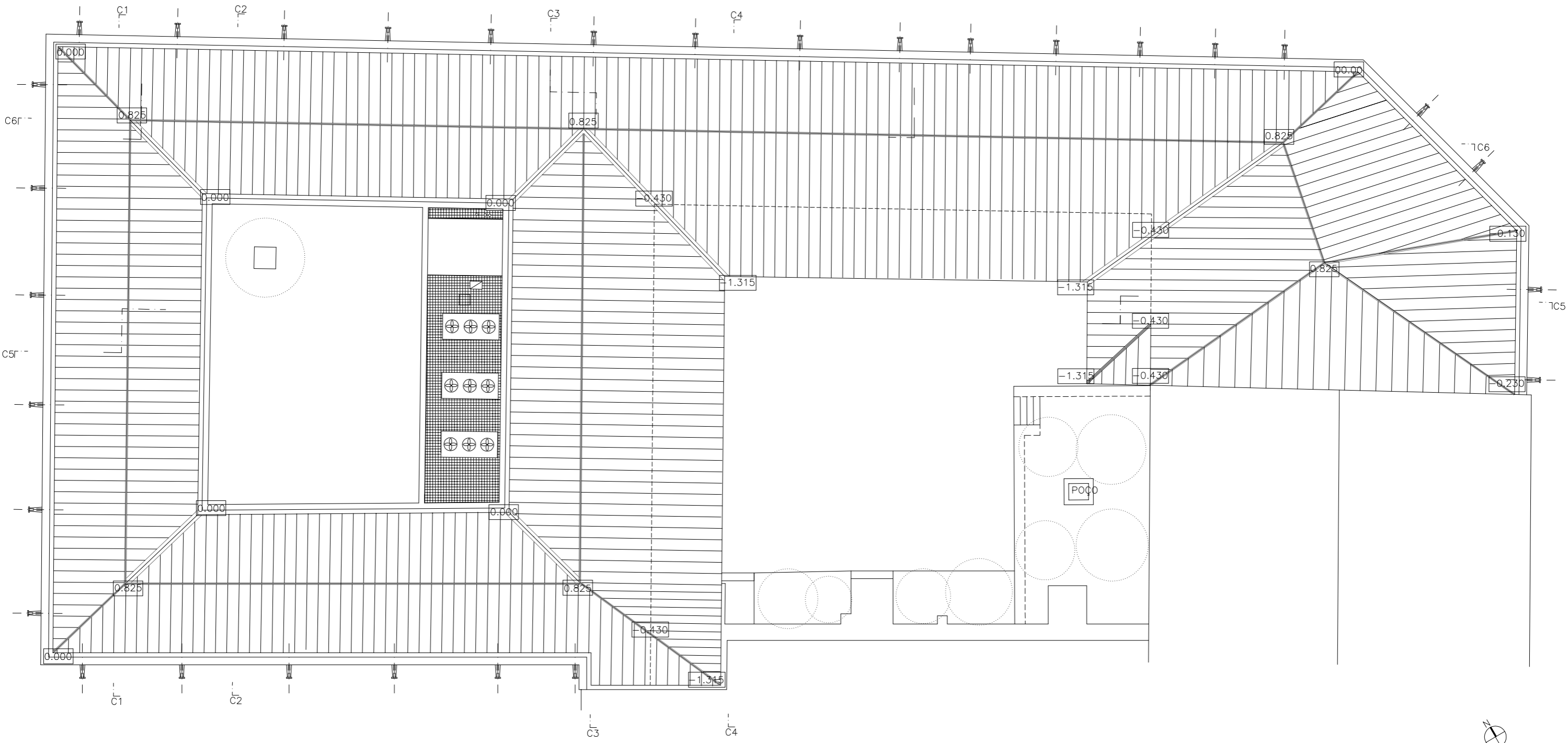
PLANTA DE COBERTURA
