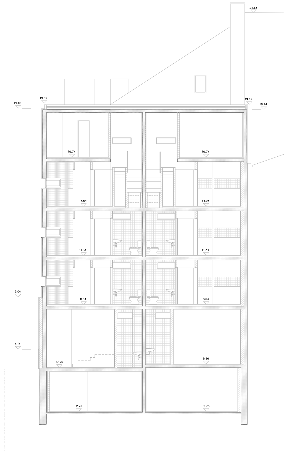
Corte GH
