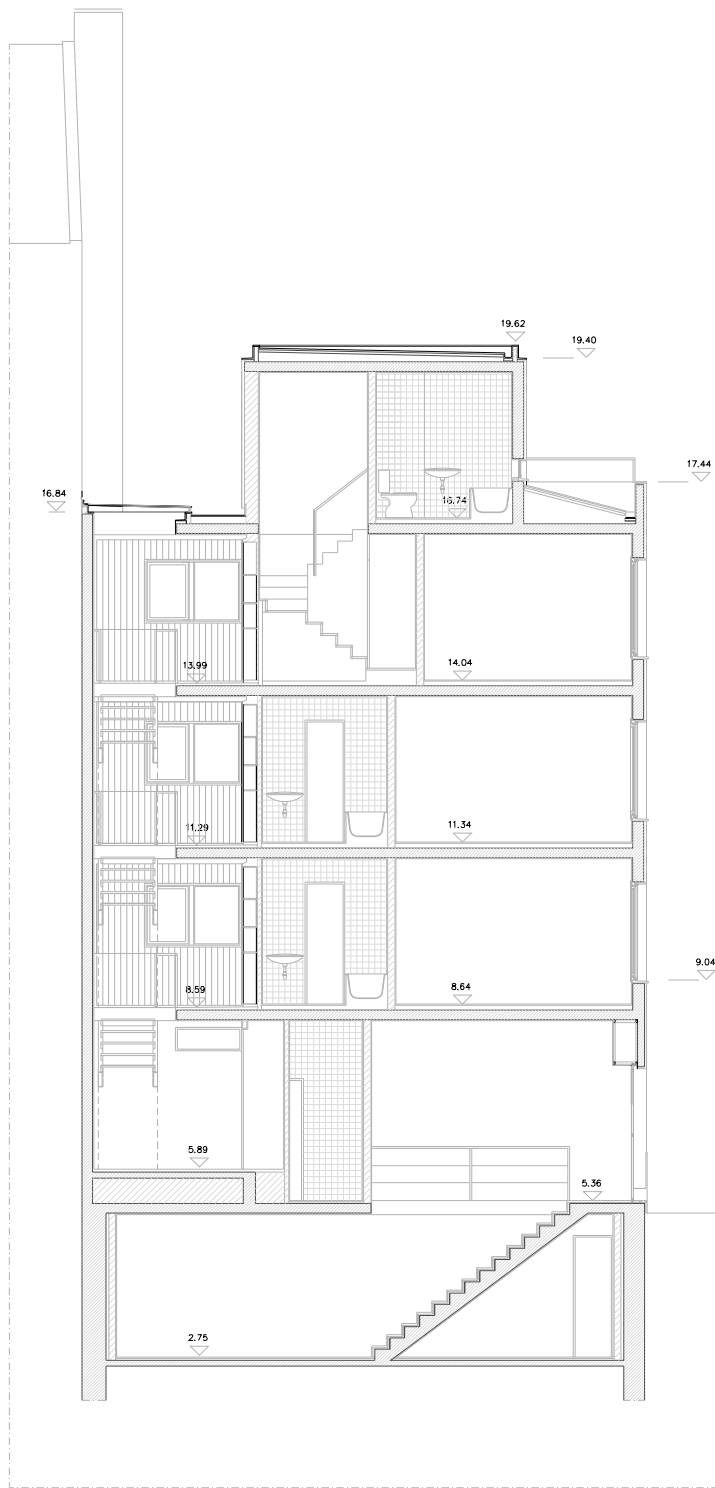
Corte CD
